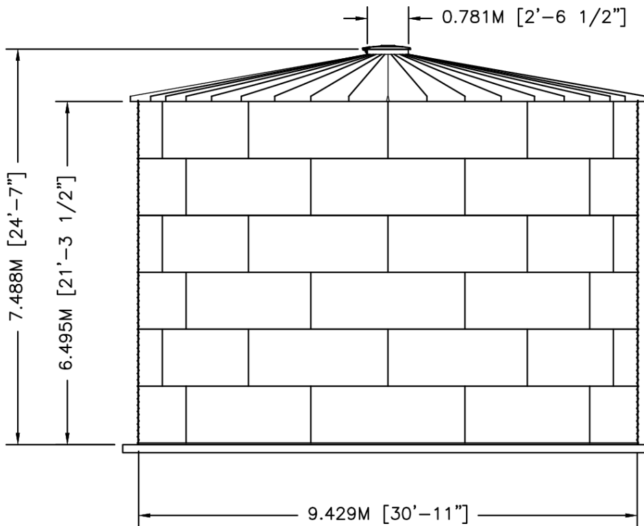
ELEVATION
